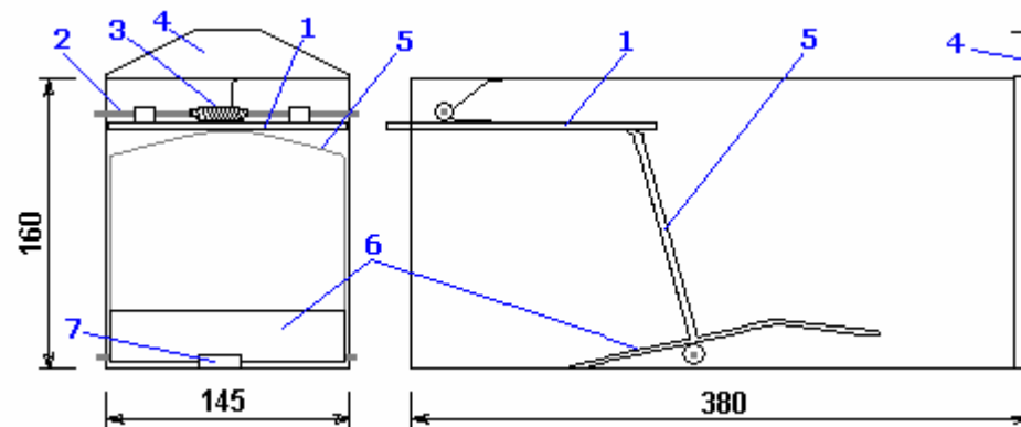
Рисунок. Живоловка в рабочем состоянии.
